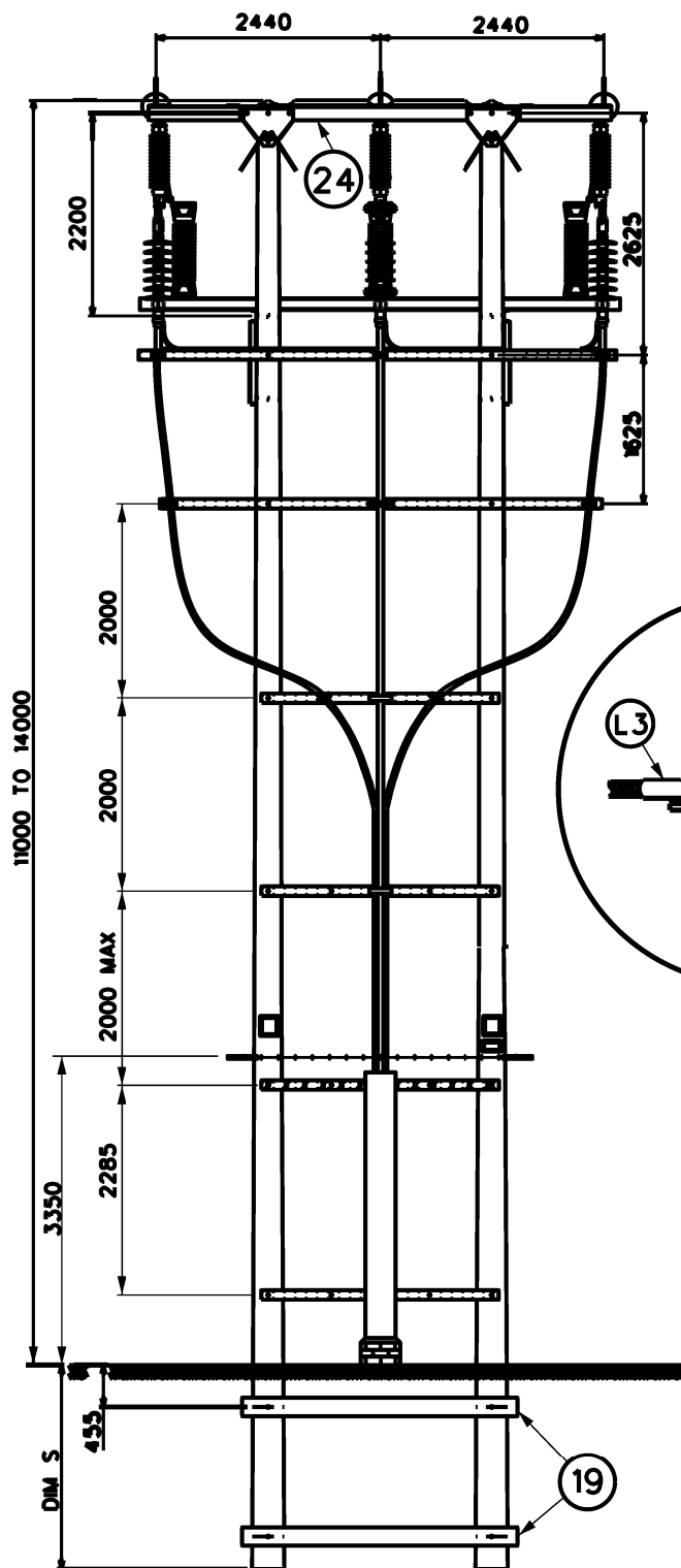
ELEVATION
